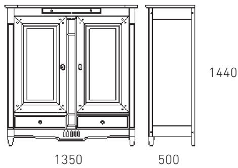
Réf MH5 Meuble d'appui 2 portes, 3 tiroirs, 1 séparation intérieure et 4 étagères.
