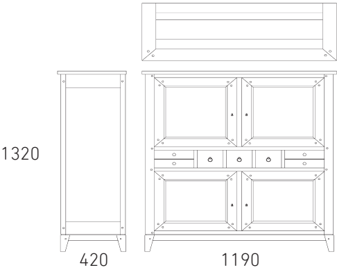
Réf FA3 Meuble de bistrot 4 portes battantes, 3 tiroirs.
