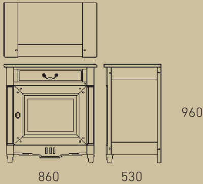
Réf MH24 Confiturier 1 porte et 1 tiroir, serrure à gauche, 1 étagère sur crémaillère bois.
