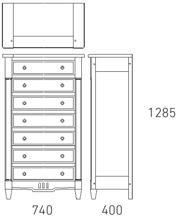
Réf MH6 Semainier 7 tiroirs.
