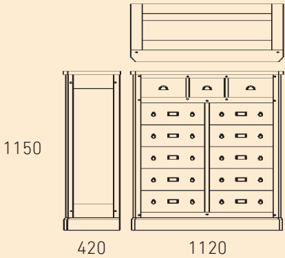
Réf FA9 Cartonnier 3 tiroirs en haut, 2 portes battantes imitation tiroirs, 1 séparation intérieure et 4 étagères.
